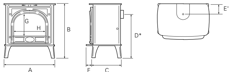
AFMETINGEN (mm) / DIMENSIONS (mm)
