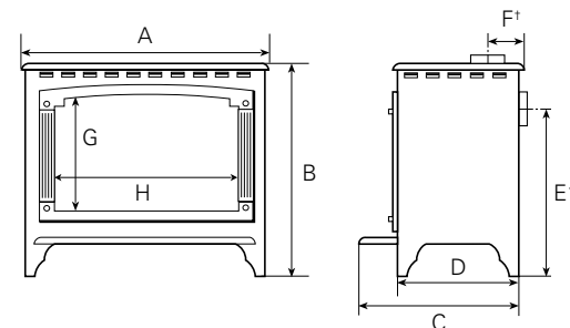
AFMETINGEN (mm) / DIMENSIONS (mm)
